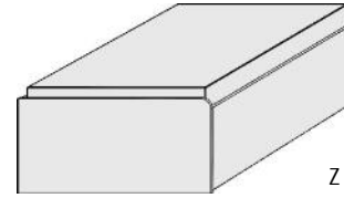
Kasten-Liege mit Doppelbettfunktion Liegefläche: 90x200cm Zusatzliegefläche: 80x190cm Zusatzbett einfach herauszieh- und hochklappbar mit 2 integrierten Metallrahmen mit Schichtholz Maßänderungen sind aufgrund der komplexen Beschlagtechnik nicht möglich
